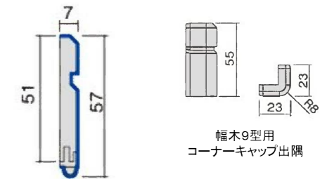
幅木9型(不陸調整用)
